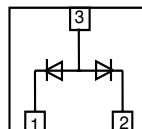
BAS70-04-HT3
