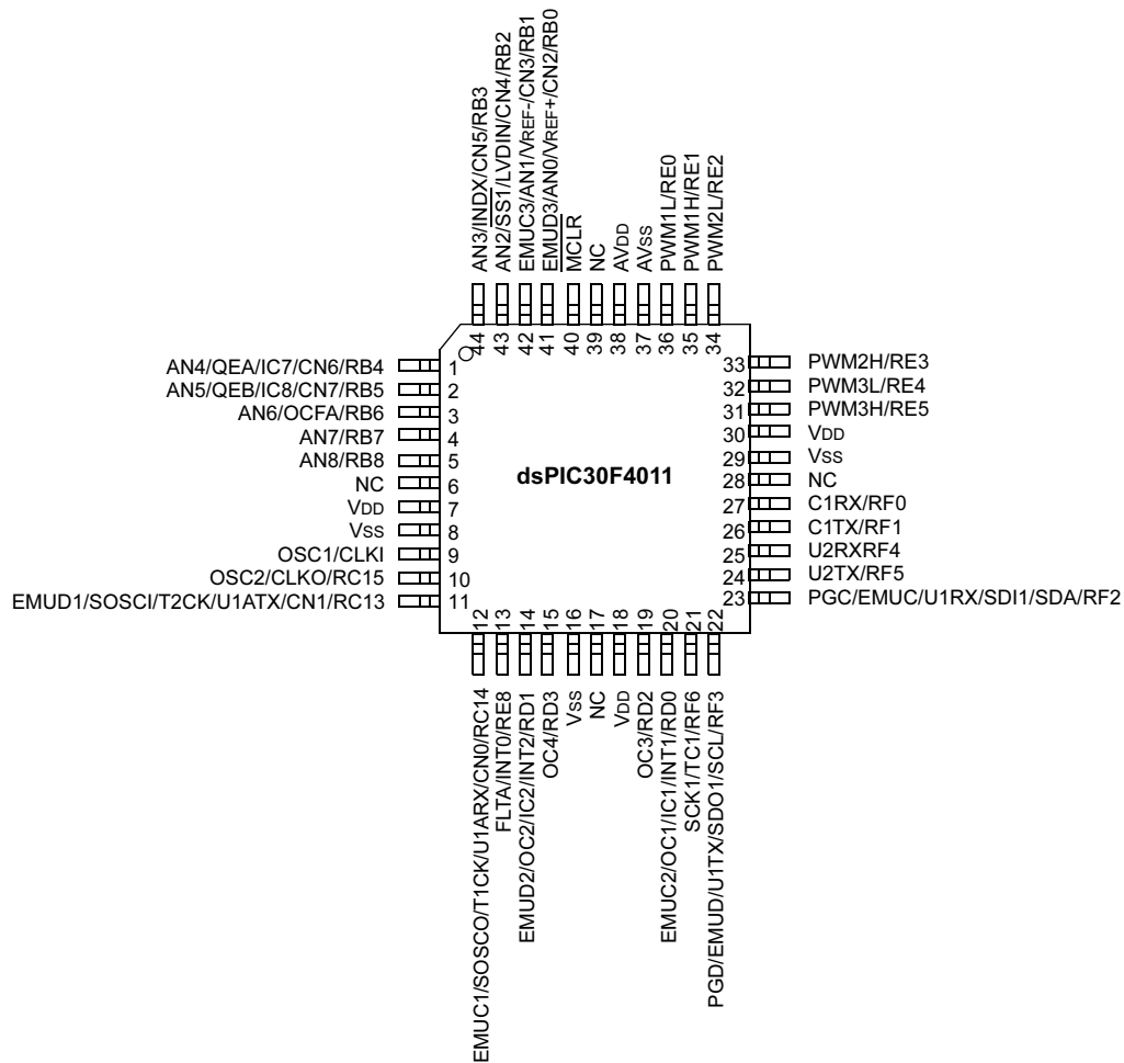
44-Pin TQFP
