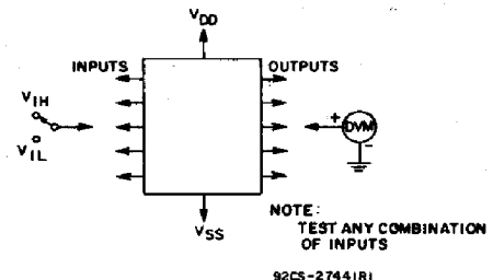
Fig. 16 - Input voltage.
