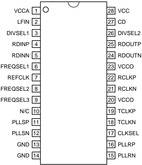
28-Pin SOIC (Z28-1) 28-Pin EPAD SOIC (S28-1)
