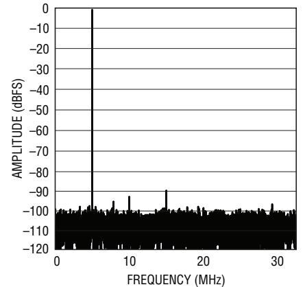
LTC2172-12: 8k Point FFT, f_{IN} = 5\text{MHz} , -1\text{dBFS} , 65\text{Mpsps}
