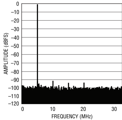
LTC2172-12: 8k Point FFT, f_{IN} = 70\text{MHz} , -1\text{dBFS} , 65\text{Mpsps}
