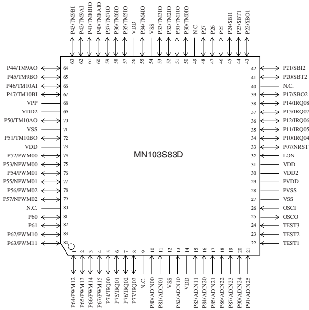
QFP084-P-1818E *Lead-free
