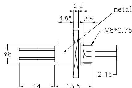
FC Receptacle
