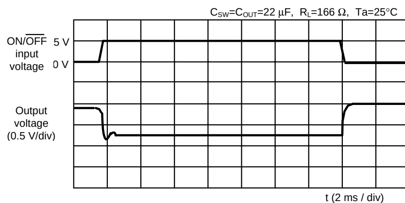
10.6 V_{IN}=7\text{ V} , SEL1=L, SEL2=H
