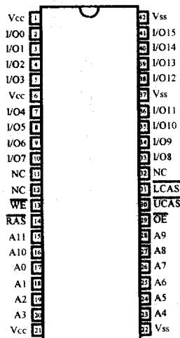
42 SOJ
