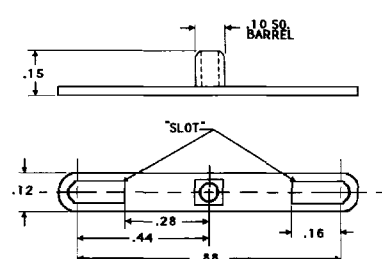
LUGS (MINIATURE)
