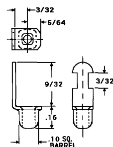
LUGS (MINIATURE)
