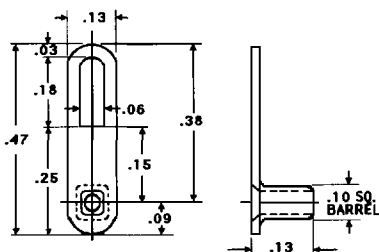
M1 LUGS (MINIATURE)
