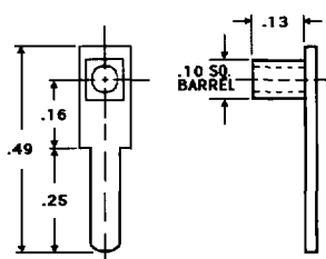
LUGS (MINIATURE)
