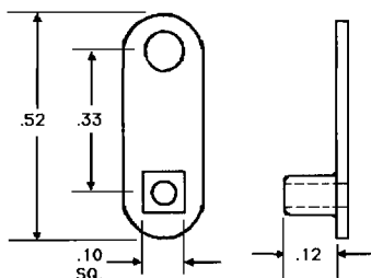
N4101 .020 BRASS MINATURE LUG
