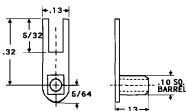
LUGS (MINIATURE)
