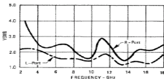
VSWR
