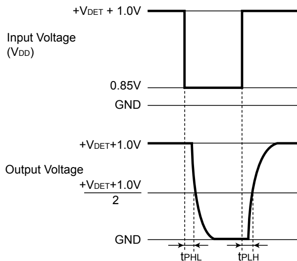
CMOS Output
