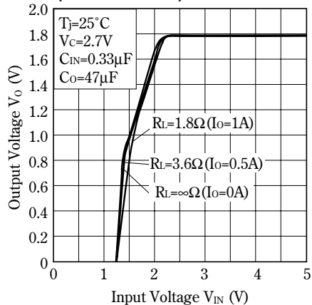
Fig.13 Output Voltage vs. Input Voltage (PQ018EF01SZ)
