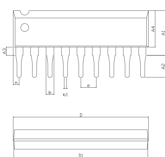
9-PIN SIP (Z09)
