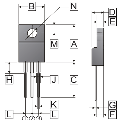
ITO-220
