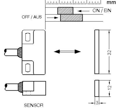
SWITCHING DISTANCES Schaltwege
