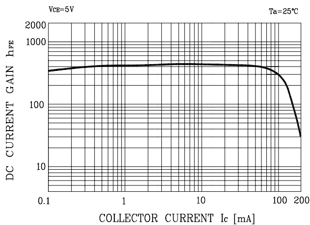
Fig. 1 h_{FE} - I_C
