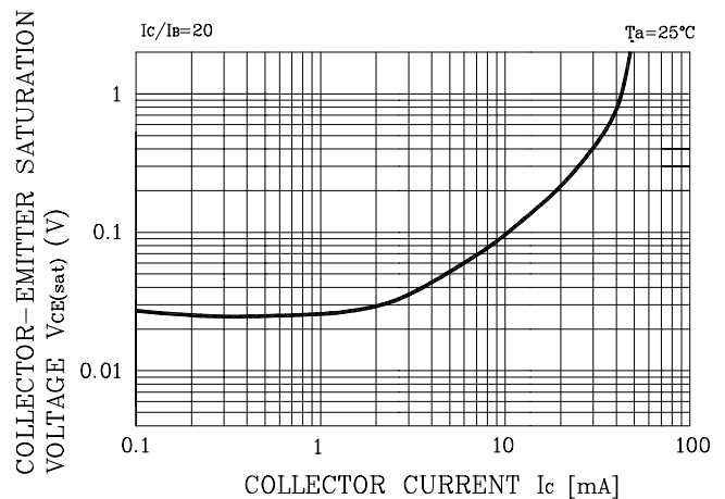
Fig. 2 V_{CE(SAT)} - I_C
