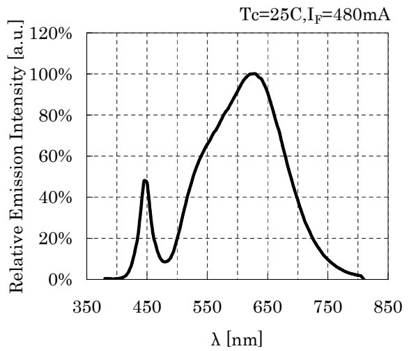
• Spectrum
