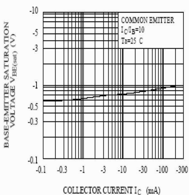
V_{BE(sat)} - I_C
