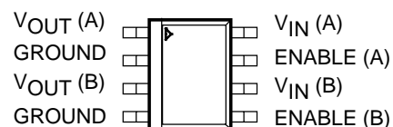
MIC5202-xxBM
