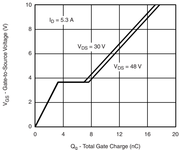
I_D = 5.3\text{ A} V_{DS} = 30\text{ V} V_{DS} = 48\text{ V} Gate Charge
