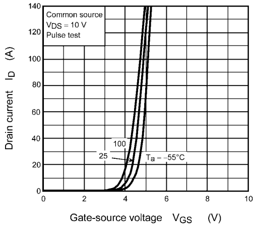
Fig. 9.3 I_D - V_{GS}
