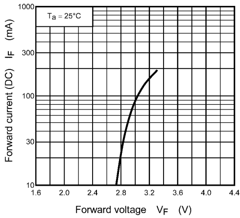
Fig. 8.1 I_F - V_F
