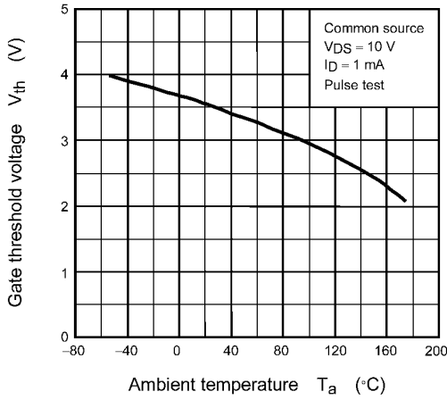
Fig. 9.9 V_{th} - T_a
