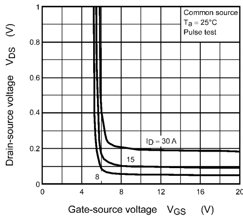
Fig. 9.4 V_{DS} - V_{GS}
