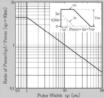
繰り返しせん頭サージ逆電力耐量 Repetitive Surge Reverse Power Capability
