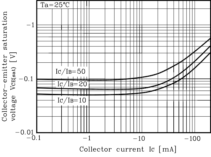
Fig. 4 V_{CE(sat)}-I_C
