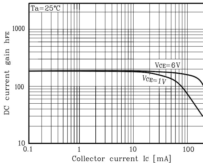
Fig. 3 h_{FE} - I_C
