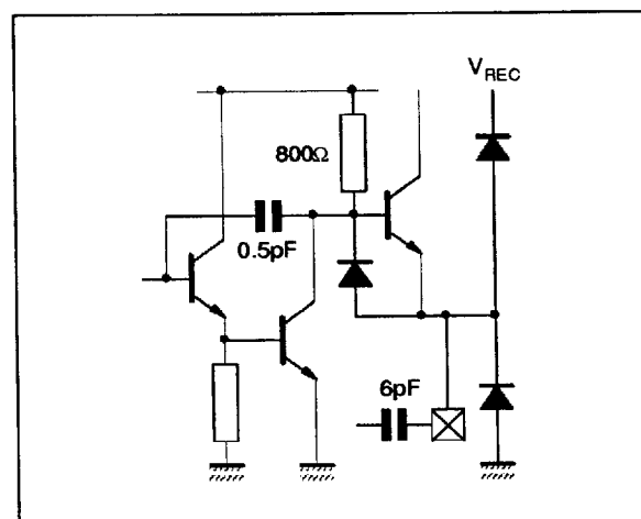
Pin : CAGC
