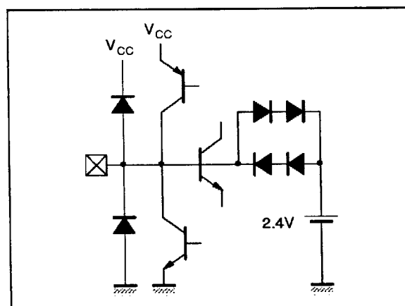
Pin : CAGC
