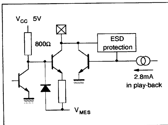
Pin : IOUT
