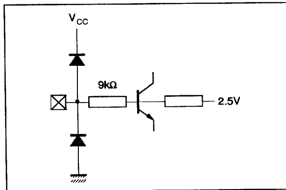
Pin : VREC
