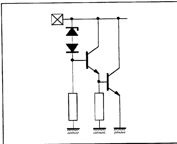
Pin : IOUT
