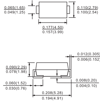
DO-214AC(SMA)
