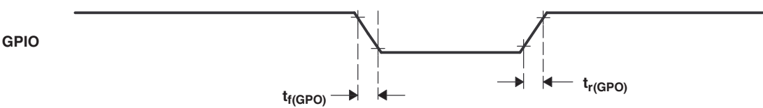
Figure 6-10. 通用输出时序
