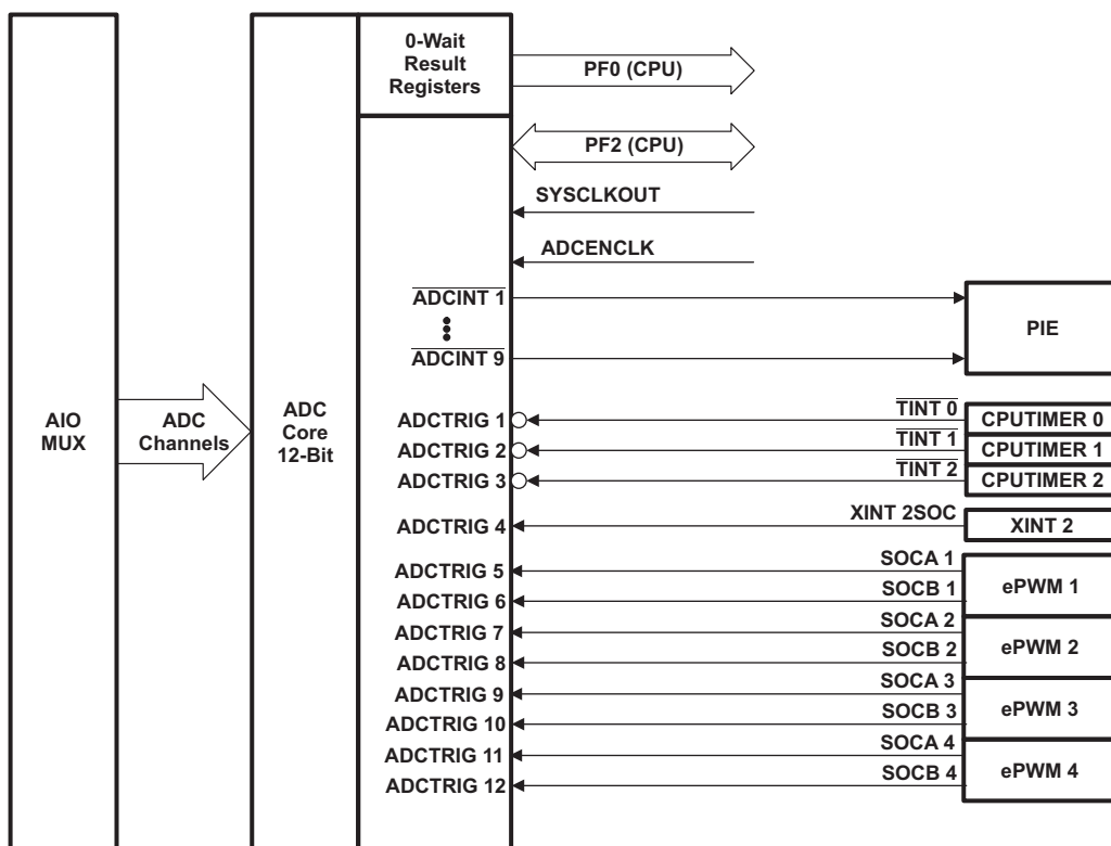
图 4-2. ADC 连接
