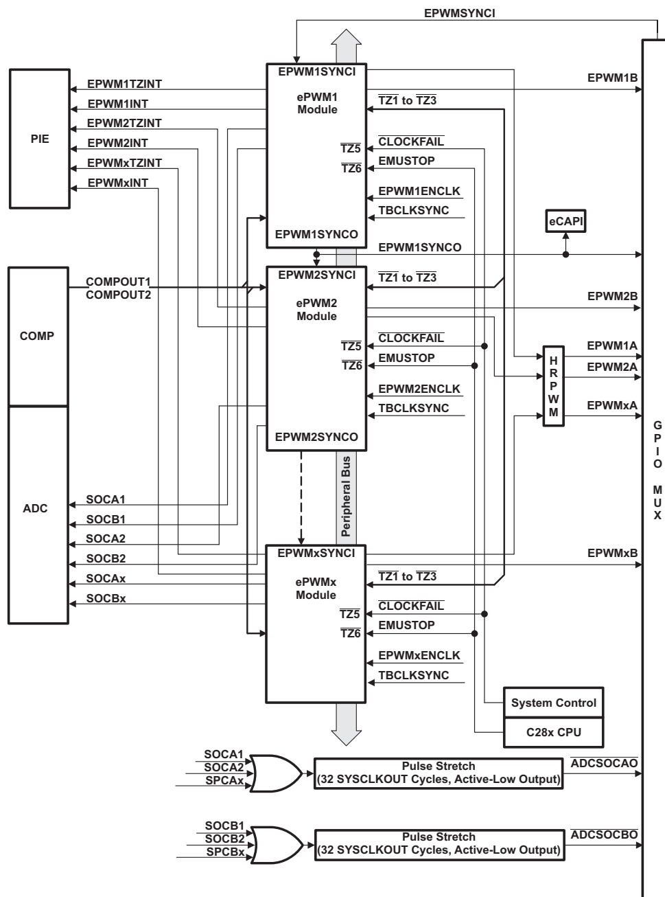
图 4-8. ePWM
