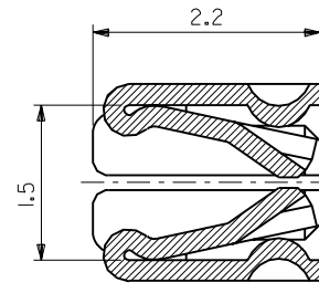
SECT. A-A (SCALE 20:1)
