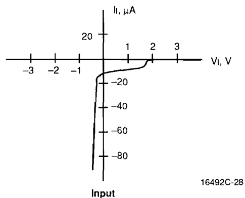
Input
