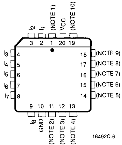
20-Pin PLCC
