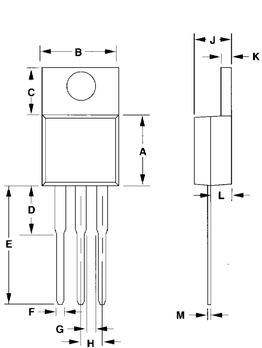
TO-220 YA Suffix
