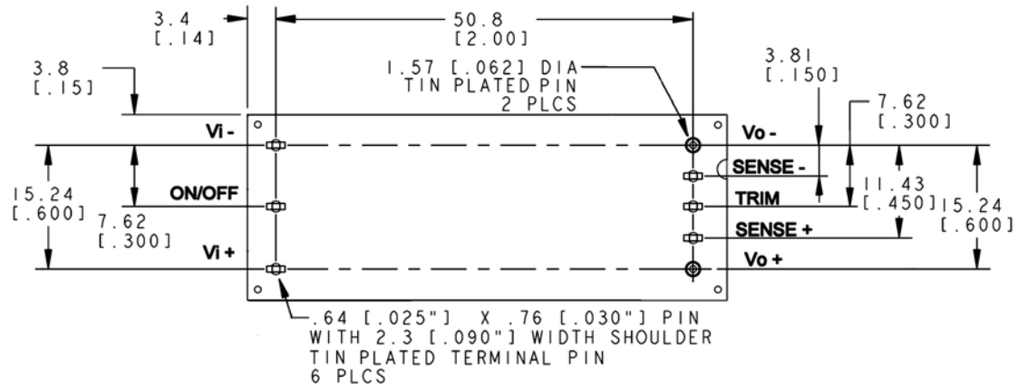
Bottom View*
