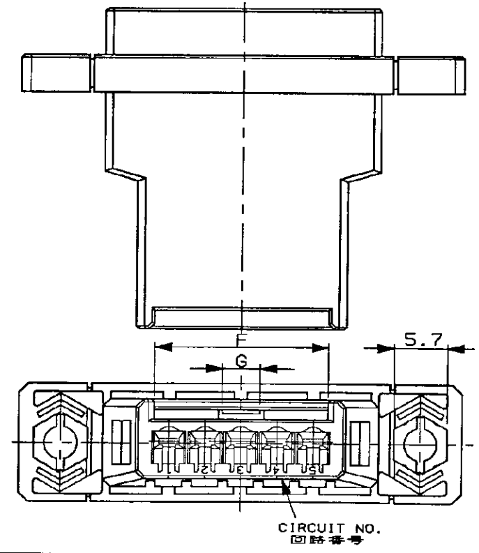
キータイプ X KEY TYPE X 1-178802-5, -7, -8
