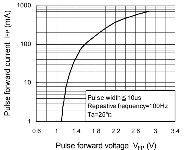
I_{FP} - V_{FP}
