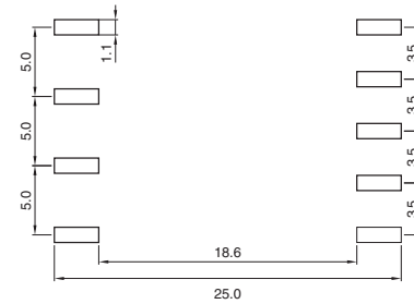
LAND PATTERNS(mm) 推奨ランド寸法
