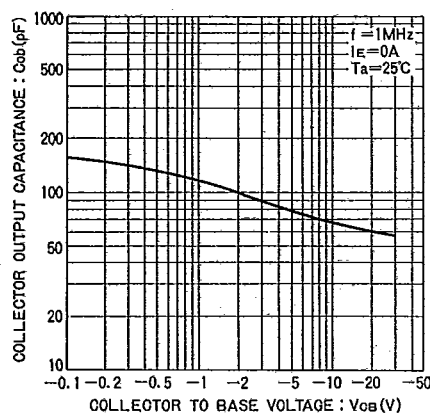
Fig.13 コレクタ出力容量 —コレクタ・ベース電圧特性
