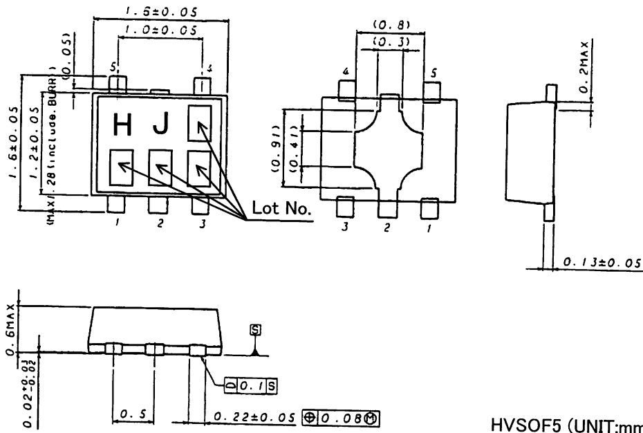
HVSO5 (UNIT:mm)
