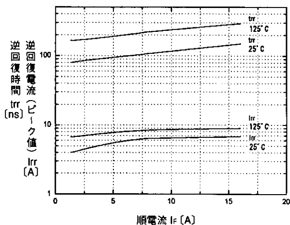
順電流 I_F (A)
