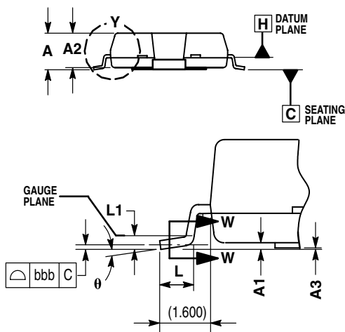
DETAIL Y
