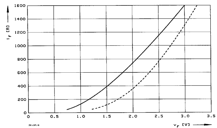
6 Durchlaßkennlinie der Inversdiode (typisch). Forward characteristic of the inverse diode (typical). --- t_{vj} = 25^\circ\text{C} , — t_{vj} = 125^\circ\text{C} , V_{GE} = 0\text{ V}
