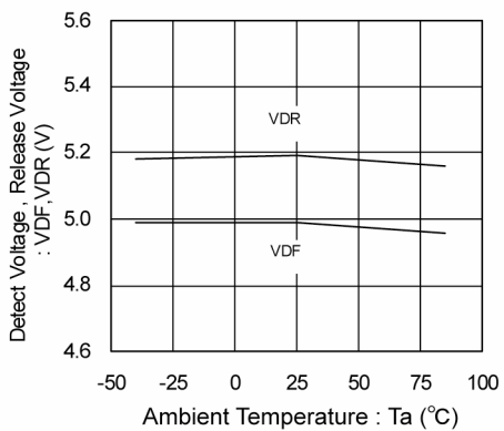
VD:5.0V
