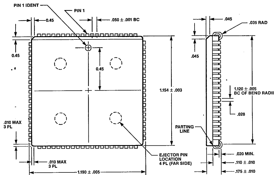
84L PLCC PACKAGE DIMENSIONS
