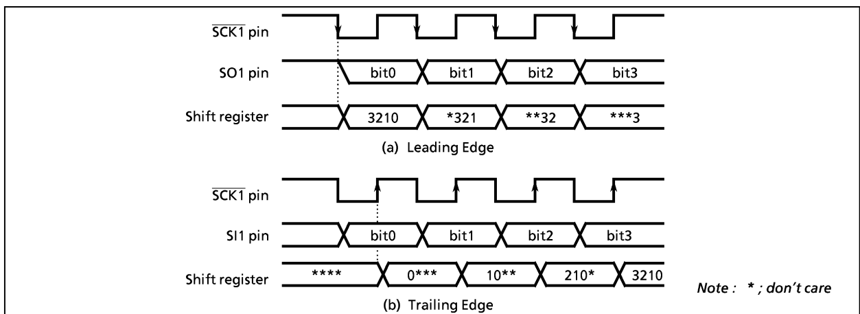
Figure 2-67. Shift Edge
