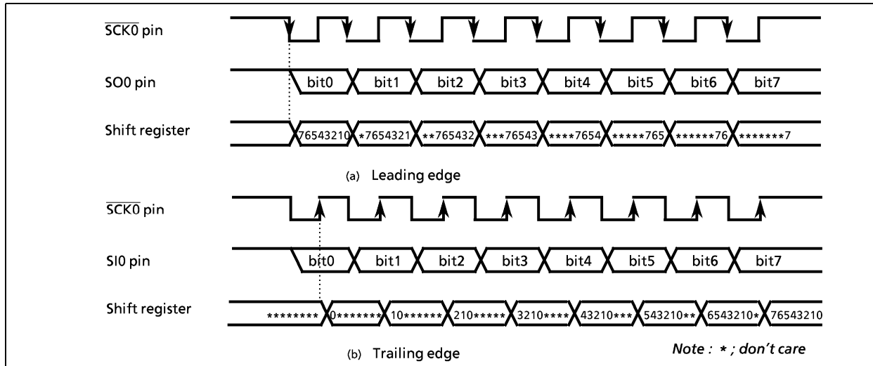
Figure 2-57. Shift Edge
