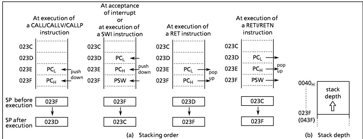
Figure 1-8. Stack
