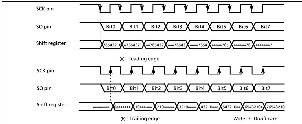
Figure 2-51. Shift Edge
