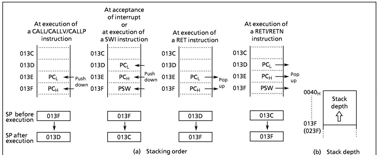
Figure 1-8. Stack
