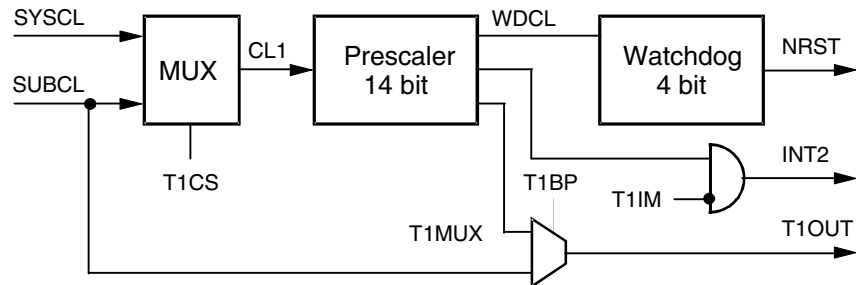
Figure 27. Timer 1 Module
