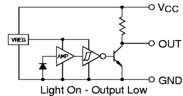
OPL536-OC Inverter/OC
