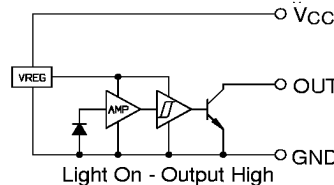
OPL535-OC Buffer/OC
