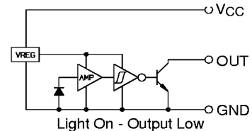
OPL536-OC Inverter/OC
