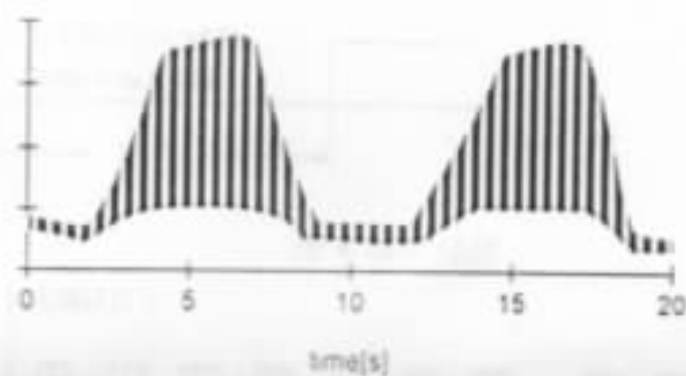
图A: 荧光灯产生的具有低频调制效应的IR信号
