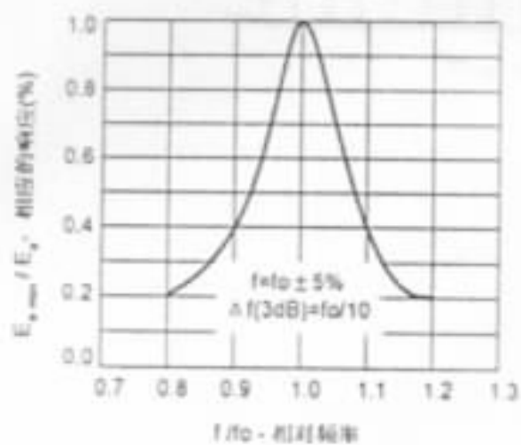
图1. 频率响应
