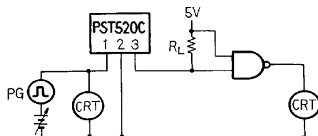
R L : 4.7k TTL IC Combination
