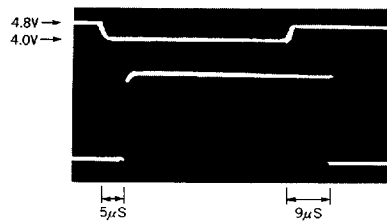
R L : 4.7k TTL IC Combination
