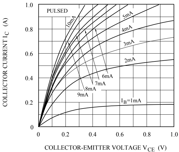
I_C - V_{CE}
